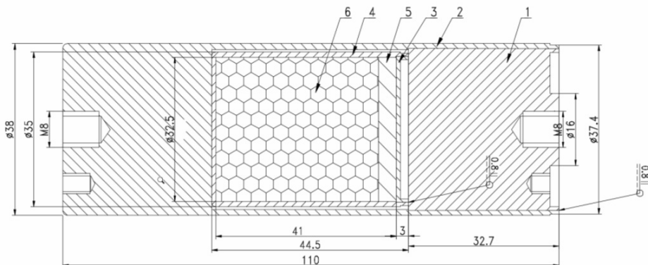
1. 外盖；2. 外包壳；3. 内盖；4. 内包壳；5. 垫块；6. 源芯 RSCSFZGCX 型特殊形式放射性物品结构示意图
